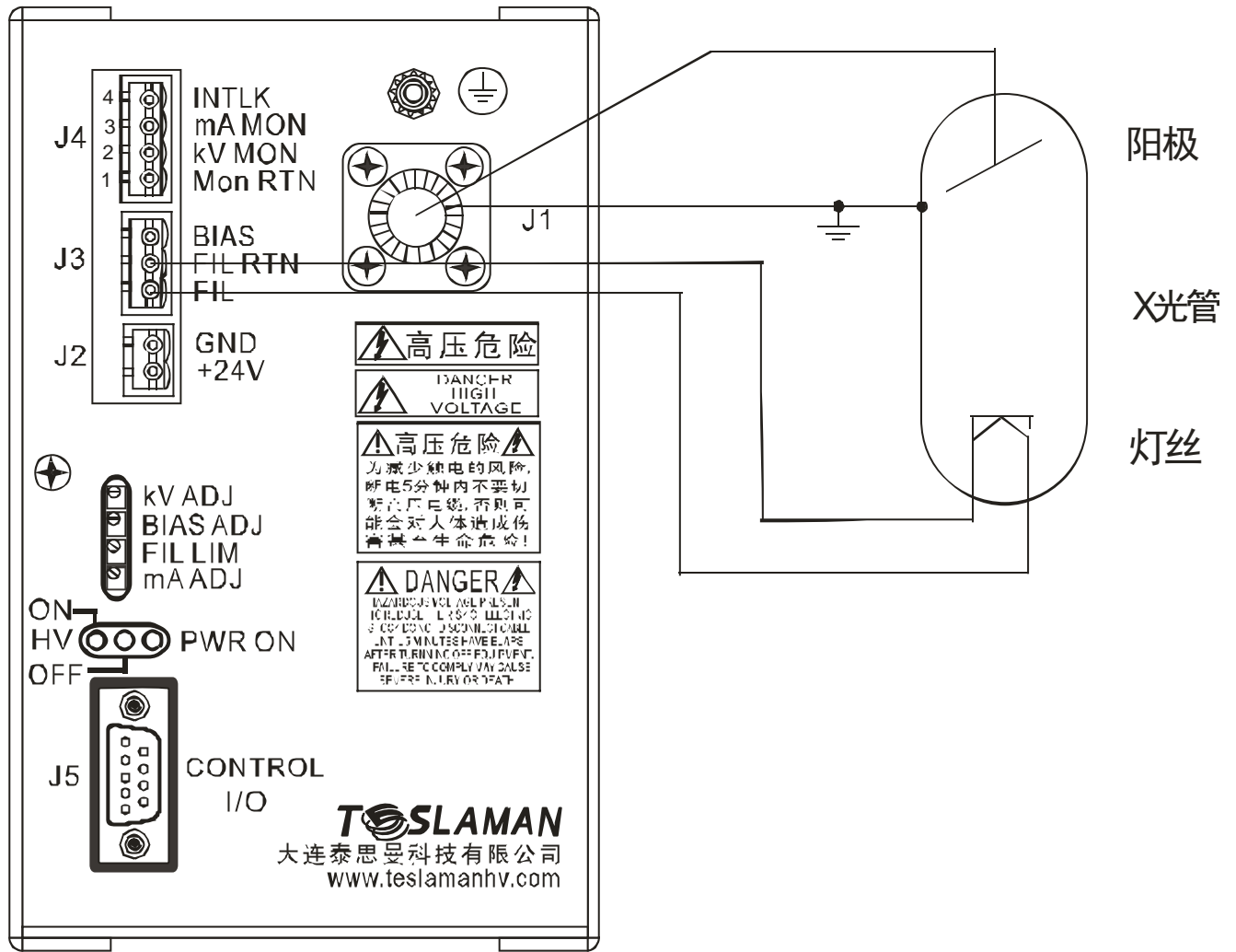
图 3.1 典型工作接线图
