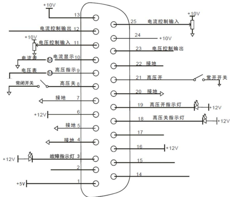
图 3.1 远程控制接线图
