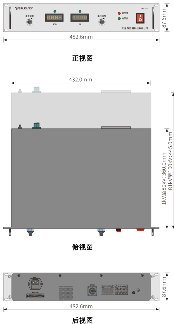
图 2.1 TRC2020 机械尺寸图
