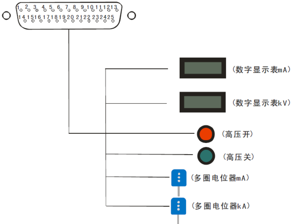
图 3.2 (2) DB25 远程控制接线图
