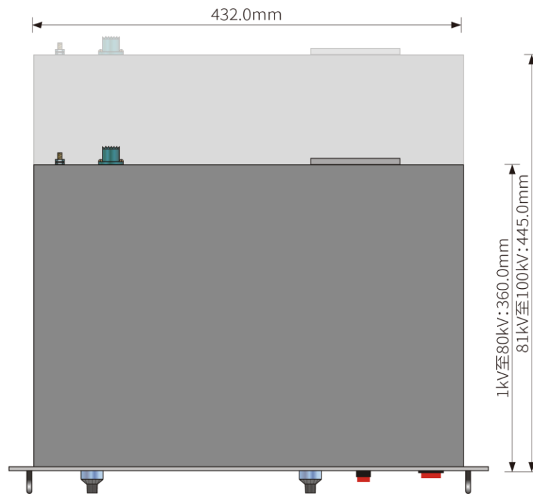
俯视图
