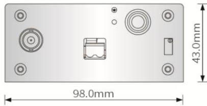
正视图
