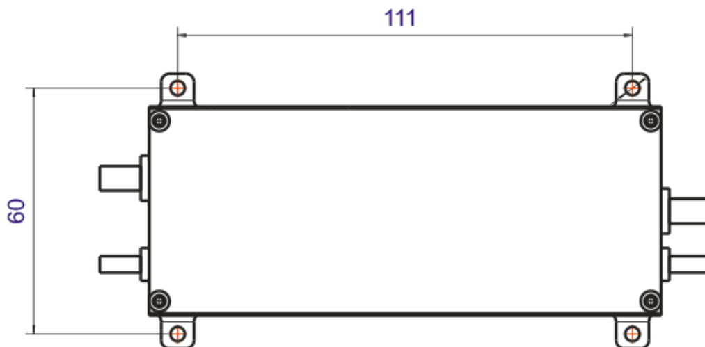
俯视图:
