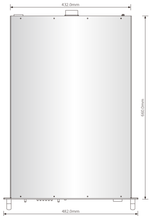
俯视图
