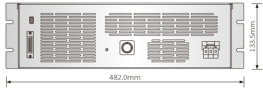
后视图
