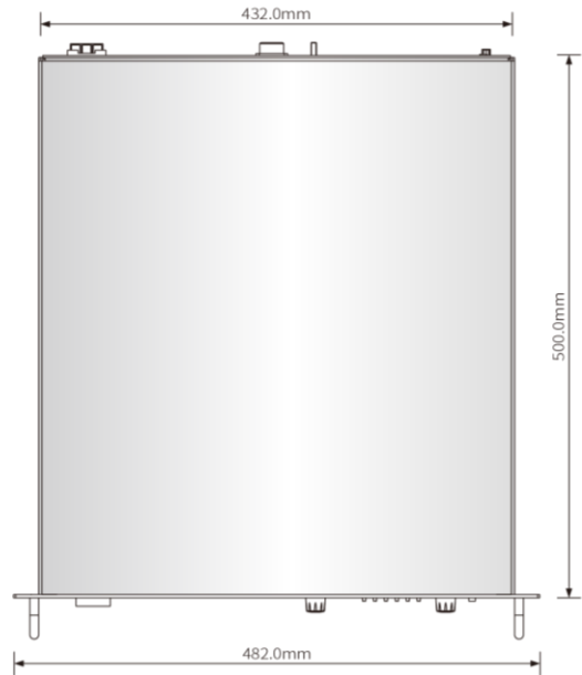
俯视图
