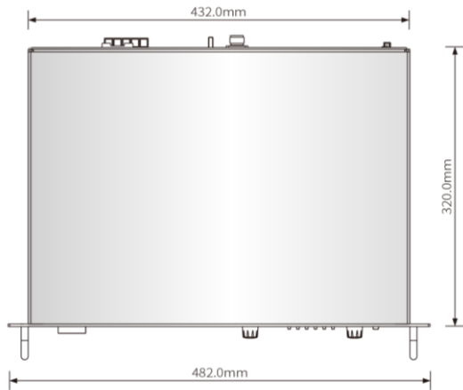
俯视图
