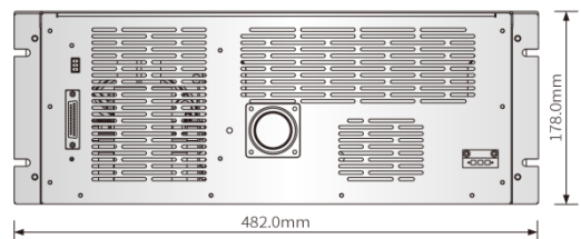
后视图
