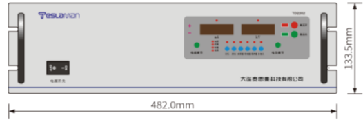
主视图
