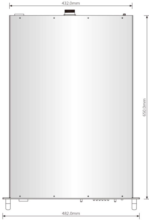
俯视图
