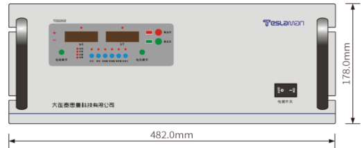
主视图
