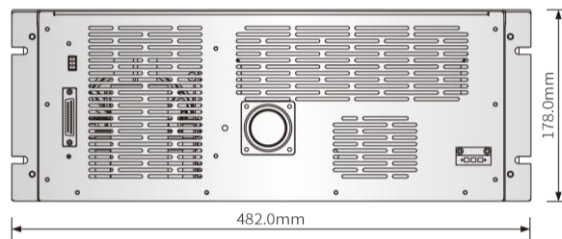
后视图
