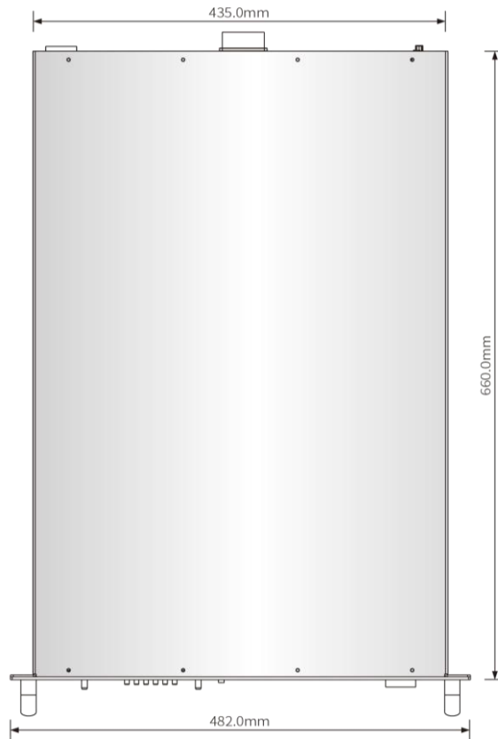
俯视图
