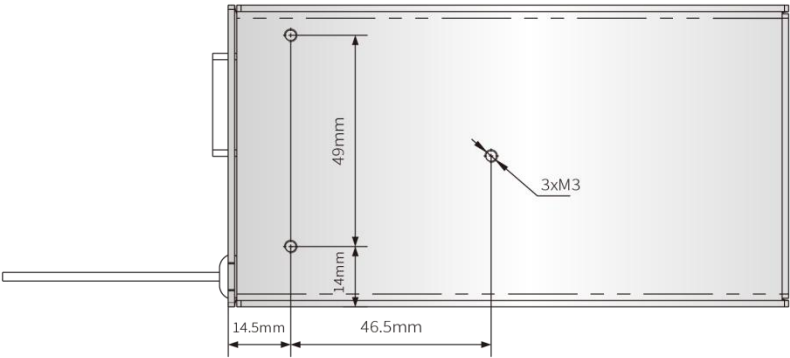
底视图
