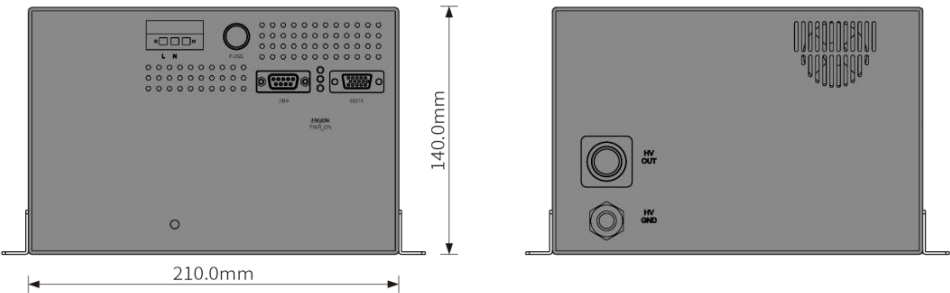
前视图
