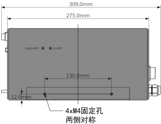
侧视图
