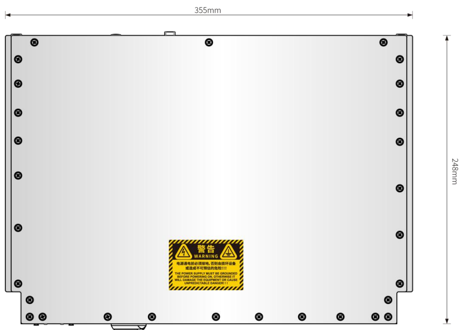
俯视图
