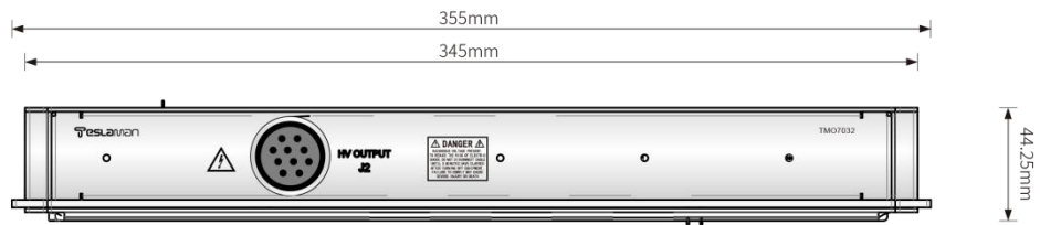
主视图
