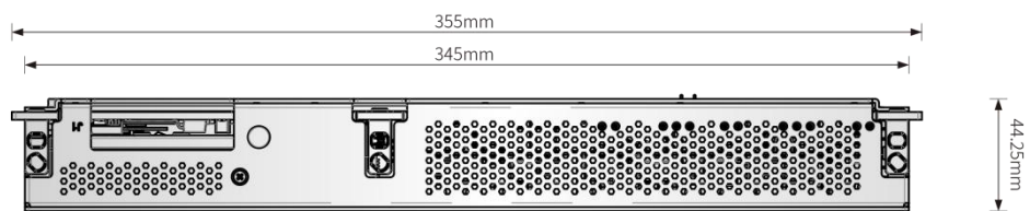
后视图
