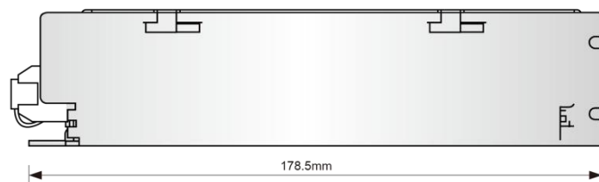
侧视图
