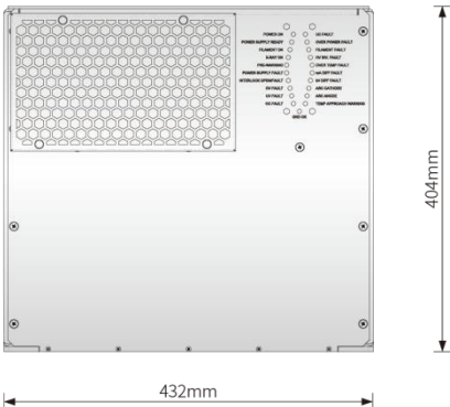
后视图
