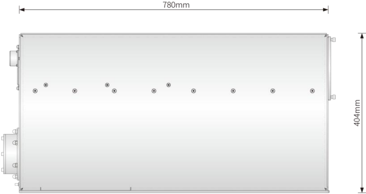
侧视图
