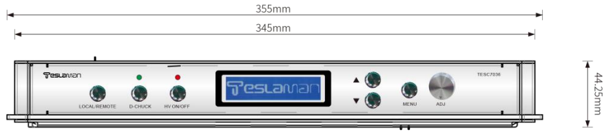
主视图
