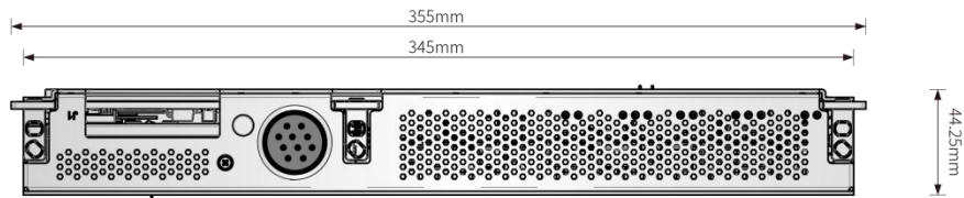
后视图
